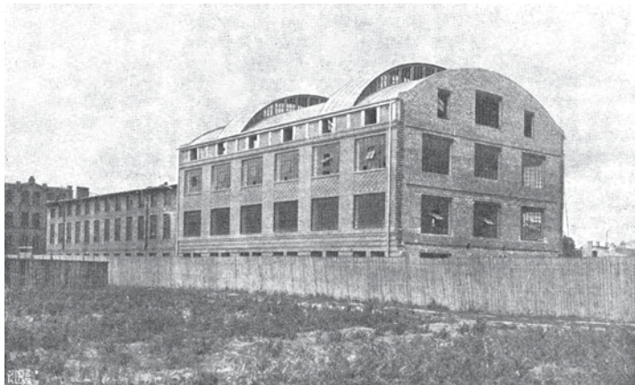
Fot. 1. Widok Fabryki Aparatów Elektrycznych K. Szpotański i Spółka S.A. od strony południowej. Po lewej stronie widać budynek niższy, tj. stary gmach fabryczny, po prawej zaś nowy gmach, który został wybudowany w 1928 roku
