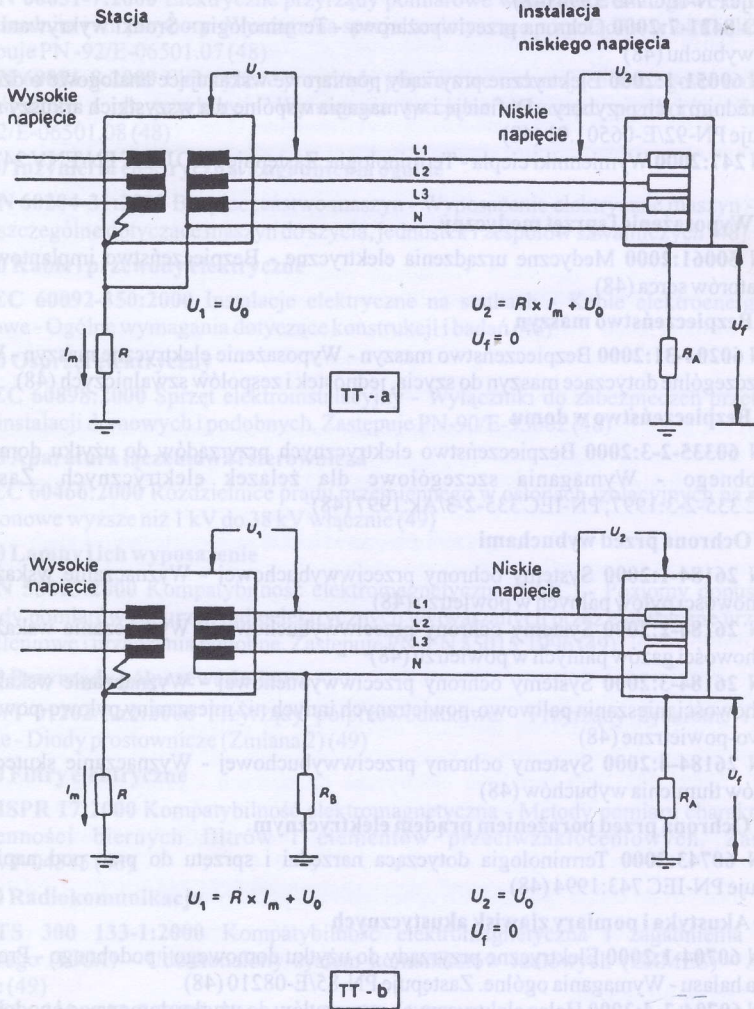
Rysunek 44 C – Układy TT
